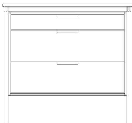
HB M0/MB 02 Modul med 3 skuffer, med eller uden bagbeklædning.
